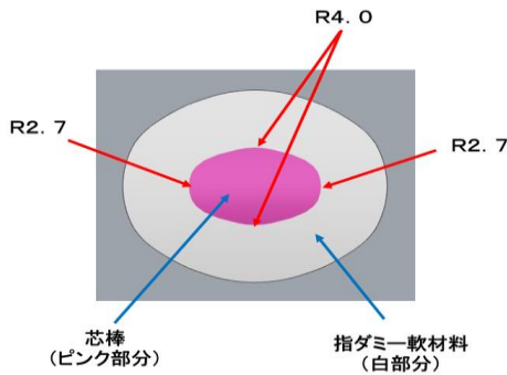
指ダミーの断面図
